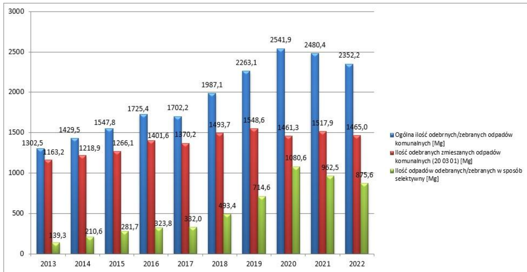
Rysunek nr 1. Ilość odpadów komunalnych odebranych/zebranych w latach 2013-2022 z wyszczególnieniem odpadów zmieszanych (20 03 01) oraz odpadów zebranych w sposób selektywny
