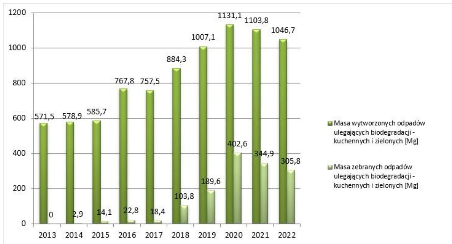
Rysunek nr 3. Ilość odebranych/zebranych odpadów komunalnych ulegających biodegradacji kuchennych i zielonych w stosunku do odpadów tego typu wytworzonych w latach 2013-2022
