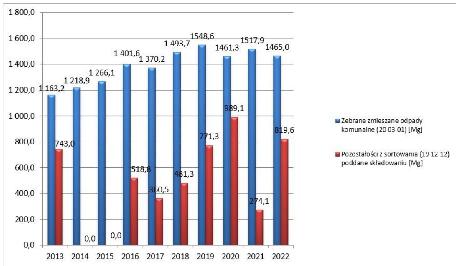
Rysunek nr 2. Pozostałości z sortowania oraz z mechaniczno-biologicznego przetwarzania odpadów komunalnych (19 12 12) poddane składowaniu w stosunku do odebranych zmieszanych odpadów komunalnych (20 03 01) w latach 2013-2022
