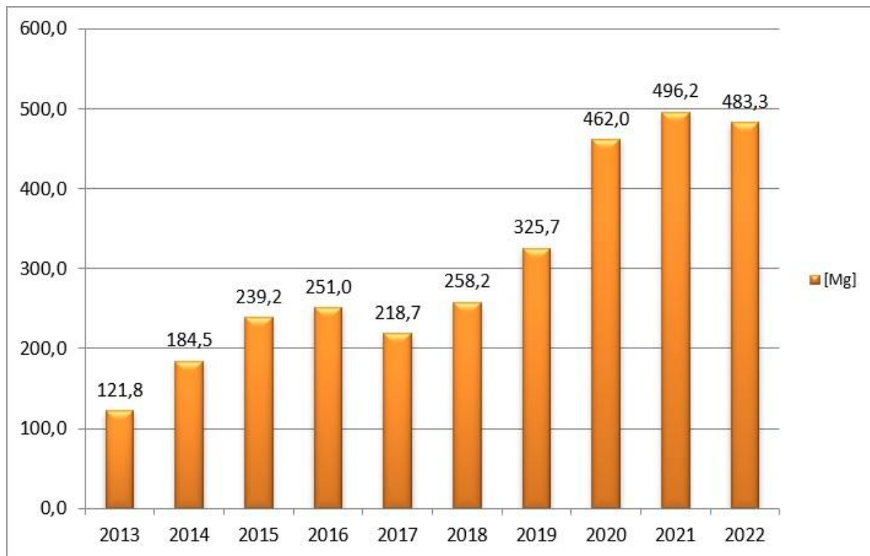
Rysunek nr 4. Ilość surowców wtórnych pochodzących z sektora komunalnego, odebranych/zebranych w latach 2013-2022
