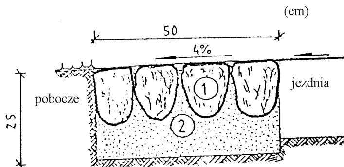
Rys. 2. Obramowanie 4-rzędowe jezdni z brukowca 1. brukowiec z kamienia łamanego lub narzutowego od 17 do 20 cm 2. ława z betonu na mokro
